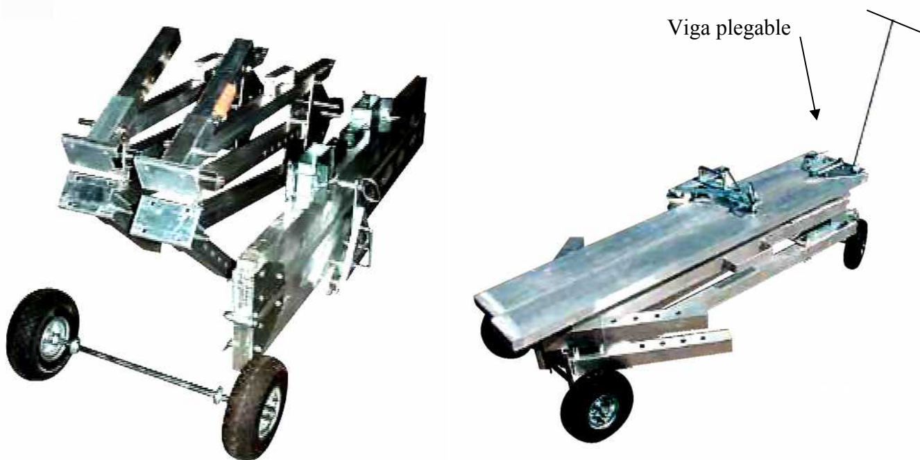
Posición de transporte
